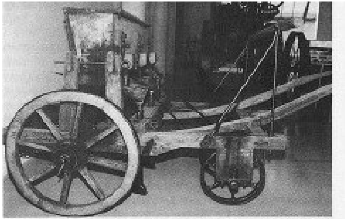
Senoir à betteraves 3 rangs PAILLARD utilisé aux environs de Pithiviers (45). Traction animale (cheval).
