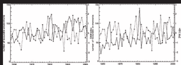
Figure 7: Variation du mode annulaire austral et du risque de CST sur la zone «WA et SA» entre 1958 et 2000.
