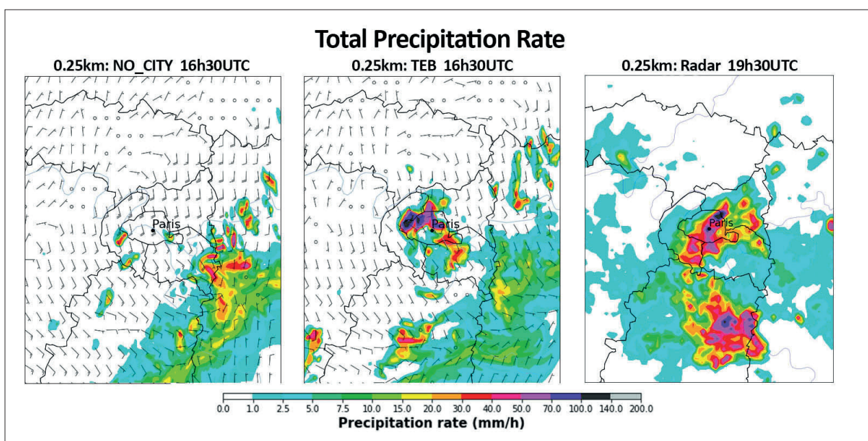
Figure 8: Taux de précipitations horaires simulées à l'échéance du maximum d'intensité au-dessus de Paris pour NO_CITY (à gauche), TEB (au milieu) et valeurs issues des réflectivités radar relevées au maximum d'intensité (à droite).
