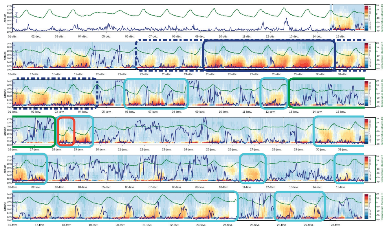
Figure 3 – Gradients de température en K/100 m calculés à partir des données du radiomètre micro-onde (couleurs chaudes pour les inversions de températures et couleurs froides pour les atmosphères instables) ; Température à 2 m en °C et vent à 10 m en m/s à la station SMC-Das (lignes verte et bleue respectivement) ; Présence de neige au sol à la station SMC-Das (flocons rouges).
