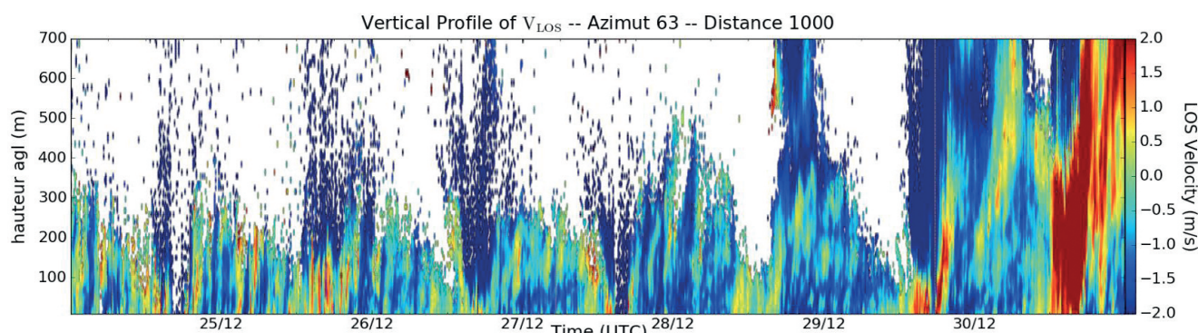
Figure 4 – Coupe verticale temporelle du vent radial (à 1000 m de SMC-Das vers le nord-est, dans la direction azimuth 63°) du 24 au 31 décembre 2016.
