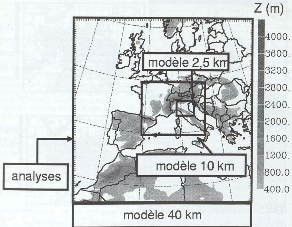
Figure 2 : schéma d'imbrication des trois modèles (résolutions horizontales respectives de 40, 10 et 2,5 km) pour la simulation numérique de la PO14. Le relief supérieur à 400 m est reporté en contours grisés.
